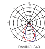
Fotometria del prodotto / Photometric curve
