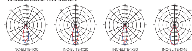
Fotometria del prodotto / Photometric curve
